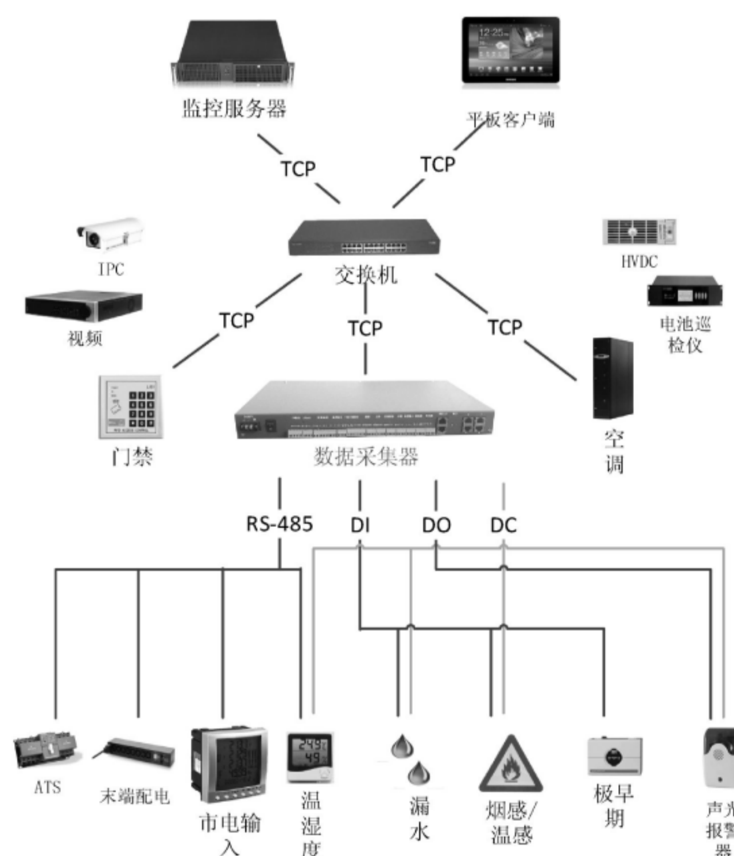
图 1 微模块管控子系统架构示意
